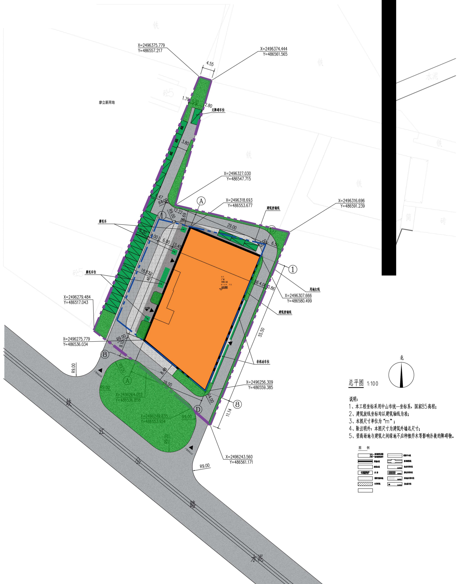
总平面图 1: 100
