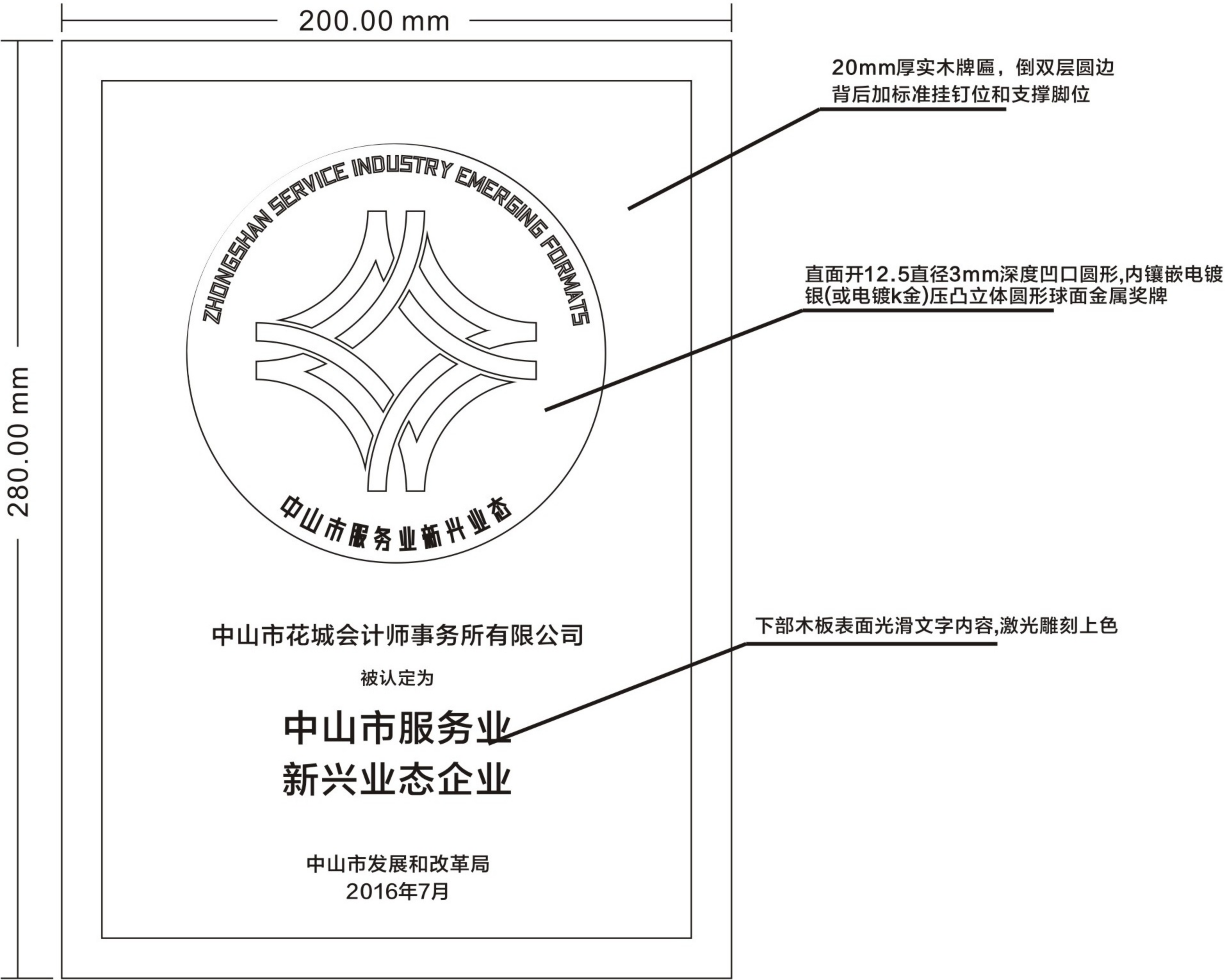
工艺示意图
