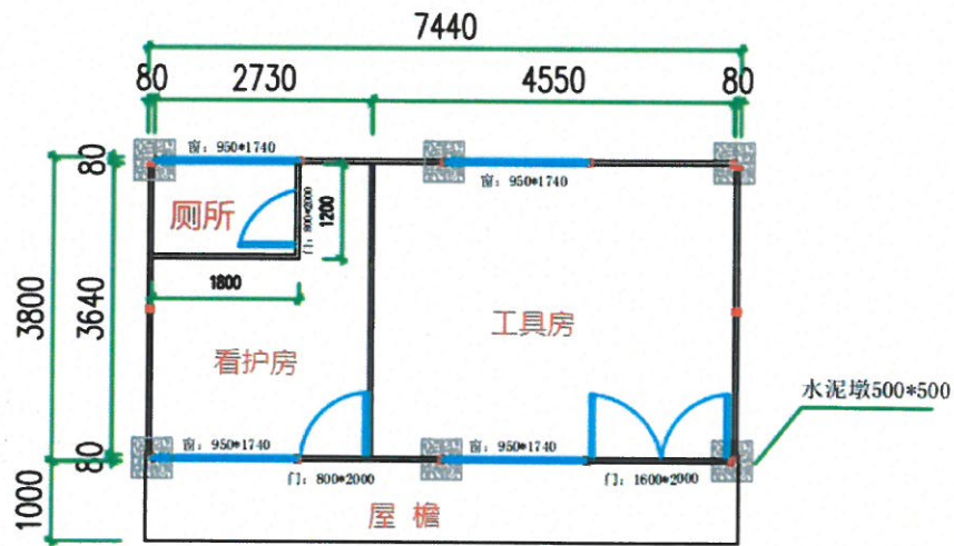
2K*4K*3P(平面图)
