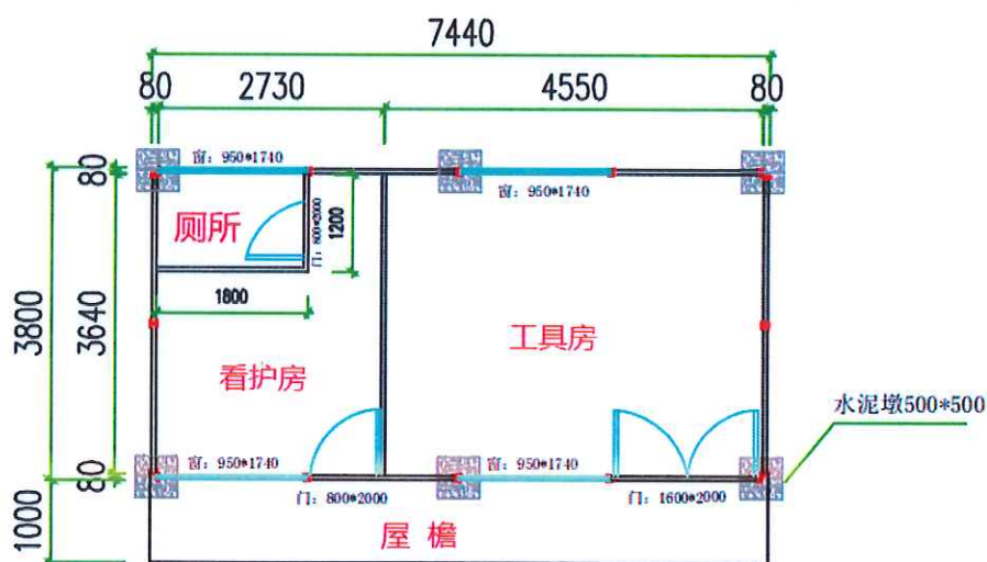
2K*4K*3P(平面图)
