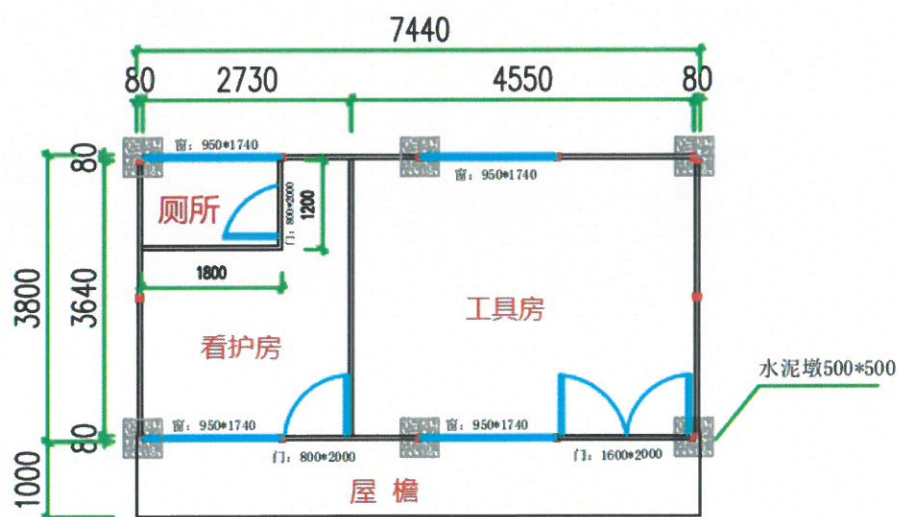
2K*4K*3P(平面图)
