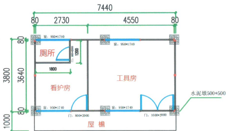
2K*4K*3P(平面图)
