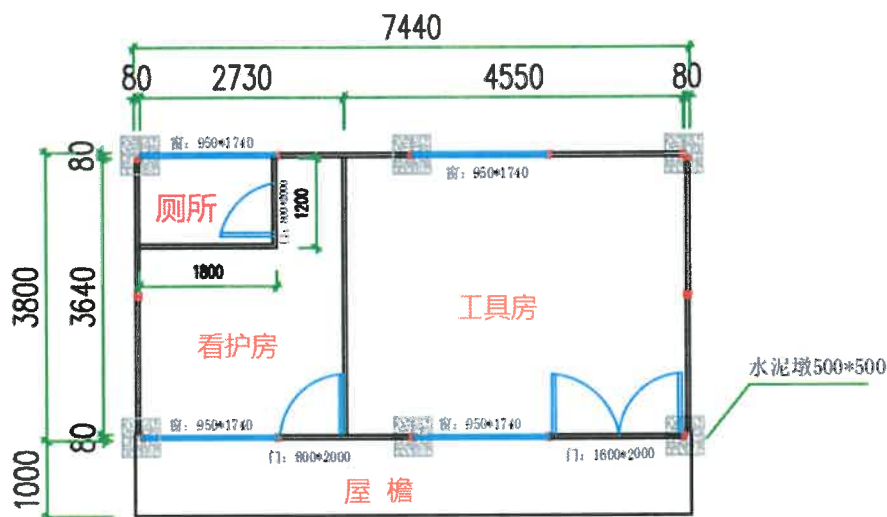
2K*4K*3P(平面图)
