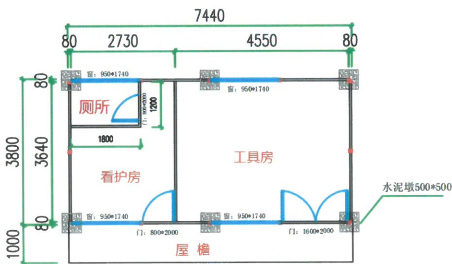
2K*4K*3P(平面图)
