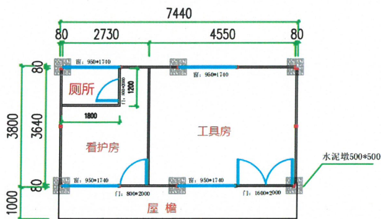
2K*4K*3P(平面图)
