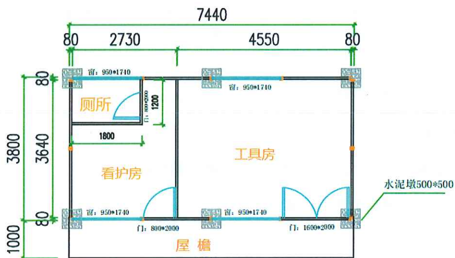
2K*4K*3P(平面图)
