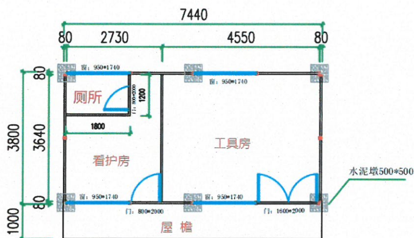
2K*4K*3P(平面图)
