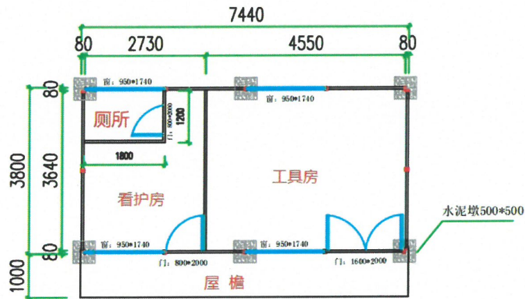
2K*4K*3P(平面图)
