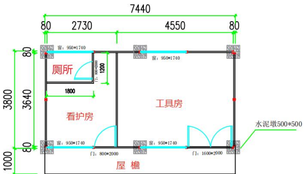
2K*4K*3P (平面图)
