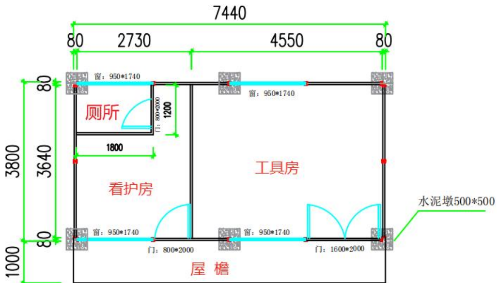
2K*4K*3P (平面图)
