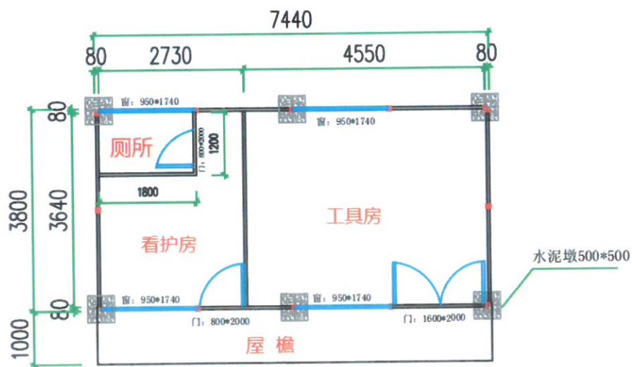
2K*4K*3P(平面图)
