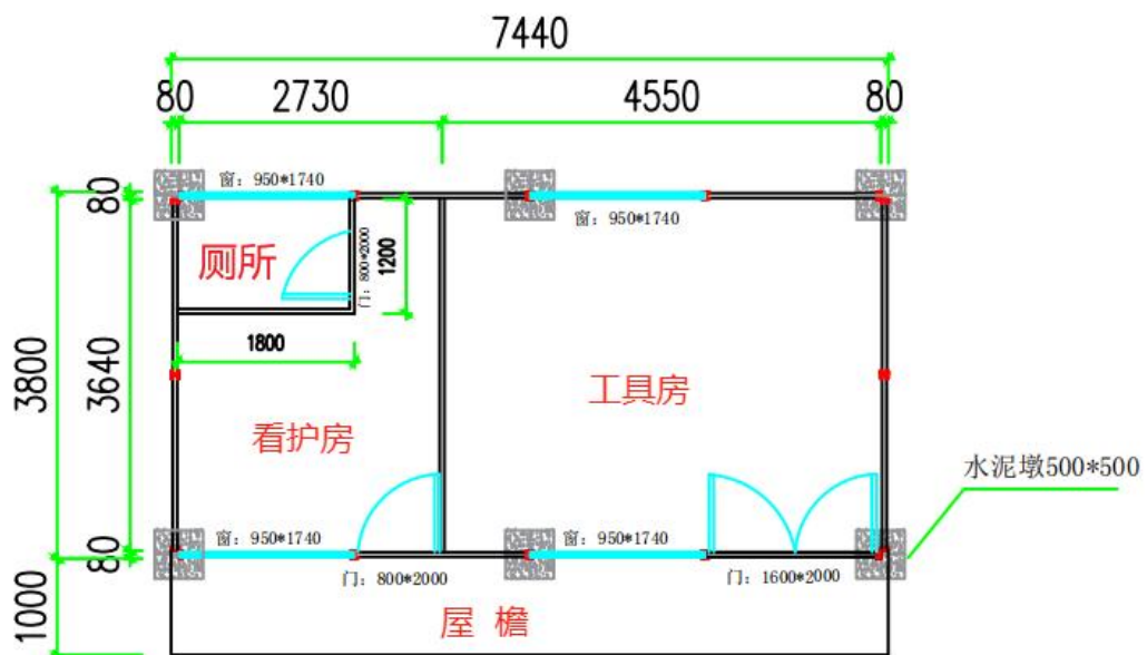
2K*4K*3P（平面图）
