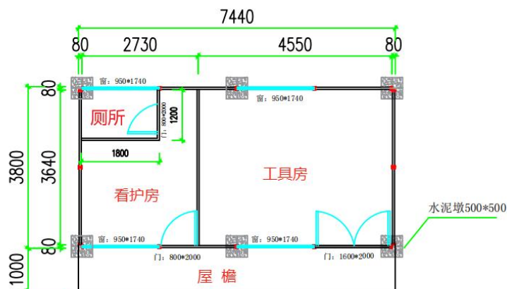
2K*4K*3P(平面图)
