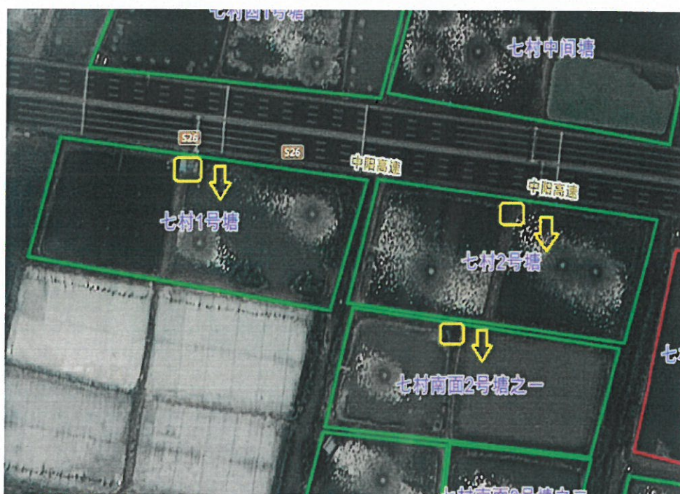
田园看护房（工具房）位置、坐向图
