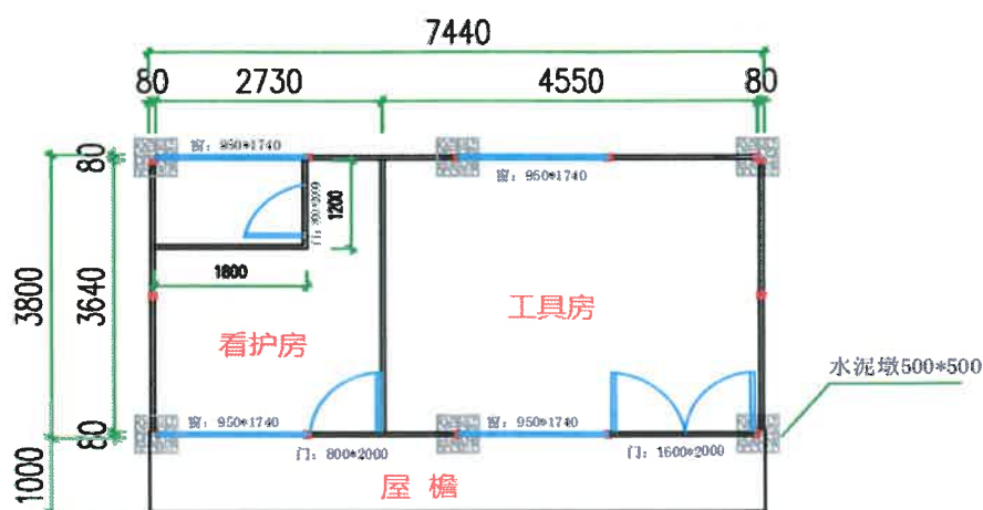
2K*4K*3P(平面图)
