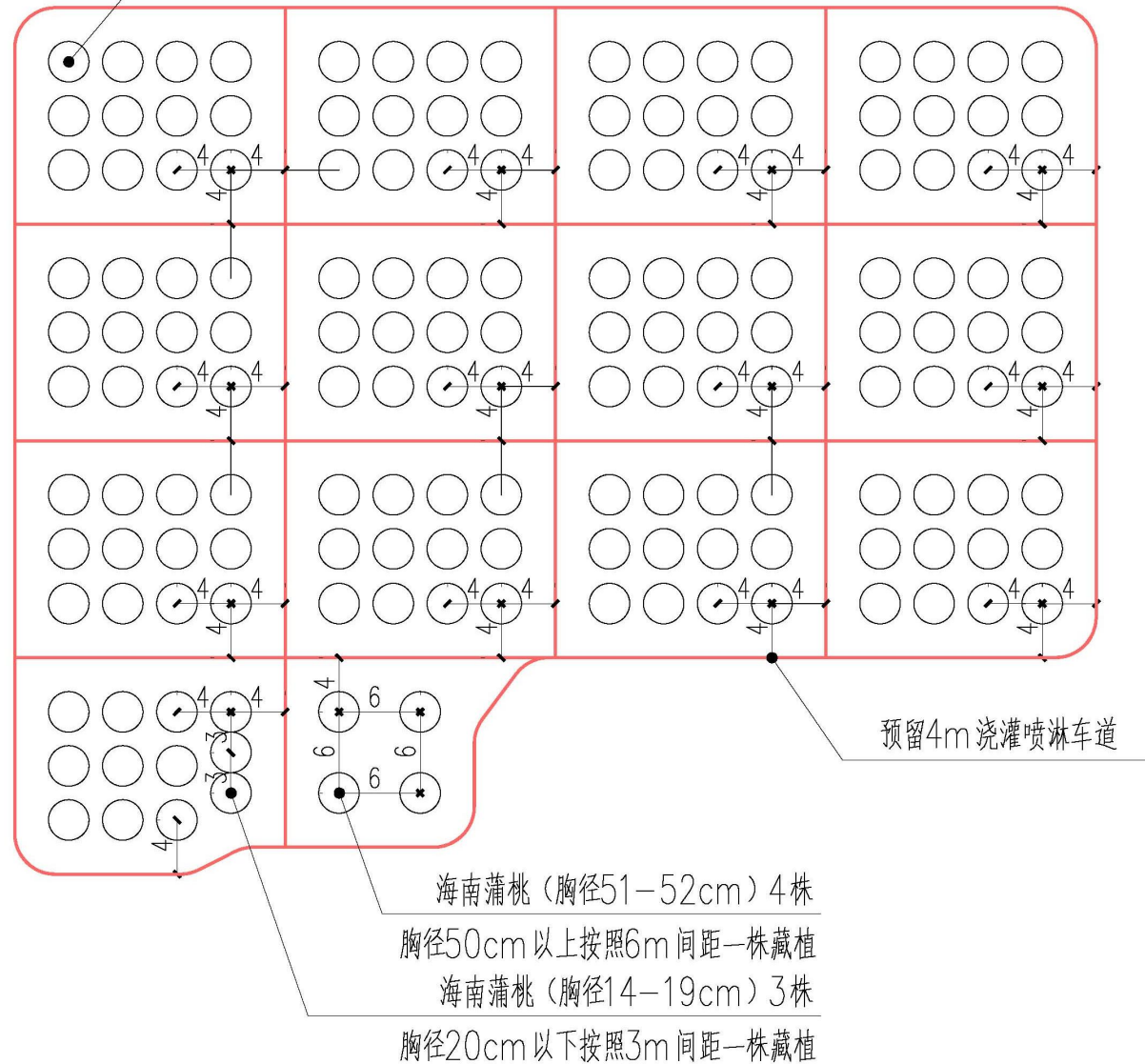
待迁移树木迁移藏植点藏植平面示意图
