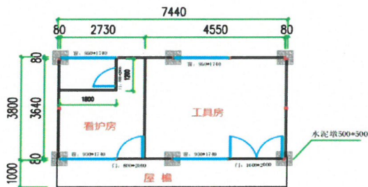
2K*4K*3P(平面图)
