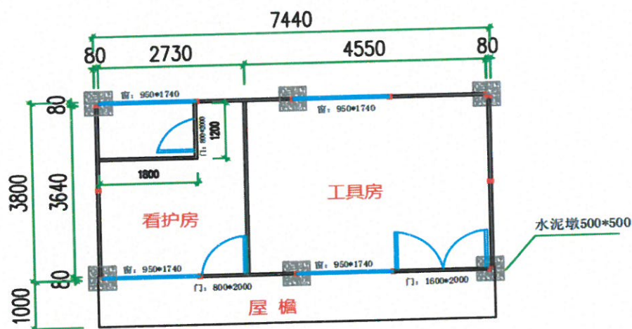
2K*4K*3P(平面图)
