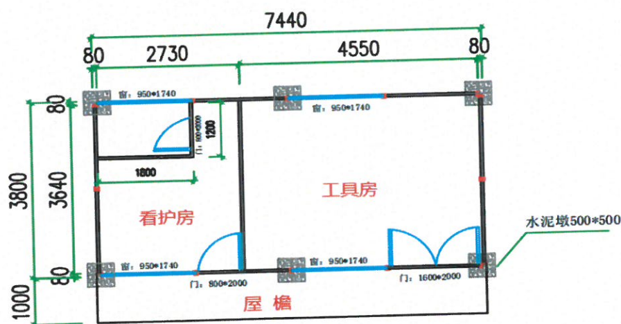
2K*4K*3P(平面图)
