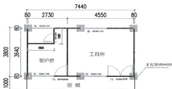
2K*4K*3P(平面图)
