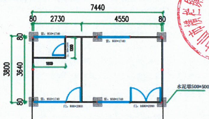
2K*4K*3P(平面图)
