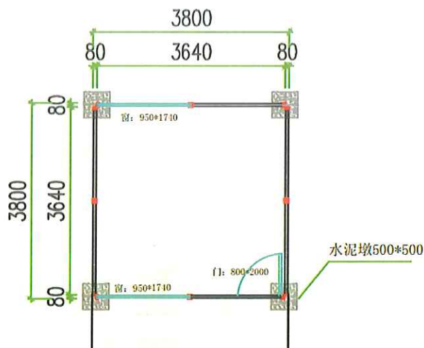
2K*2K*3P (平面图)
