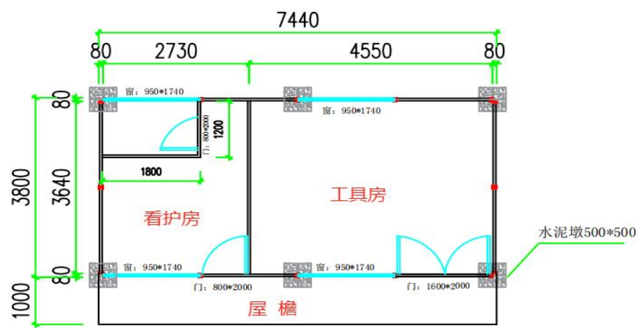
2K*4K*3P(平面图)
