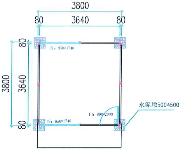
横栏镇田园看护房（工具房）样式平面图
