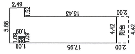
砖混结构二层平面图
