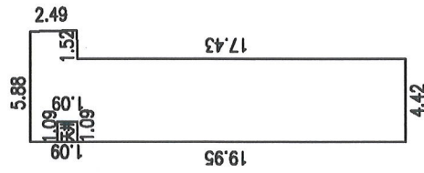
砖混结构一层平面图
