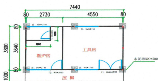
2K*4K*3P(平面图)
