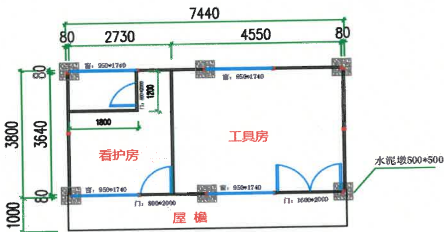
2K*4K*3P(平面图)
