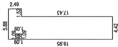
砖混结构一层平面图
