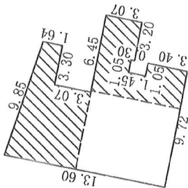
F001: 一层平面图 建筑面积: 124.45m²
