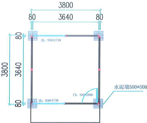
2K*2K*3P (平面图)
