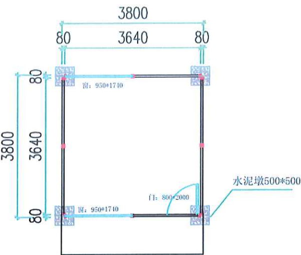
2K*2K*3P (平面图)
