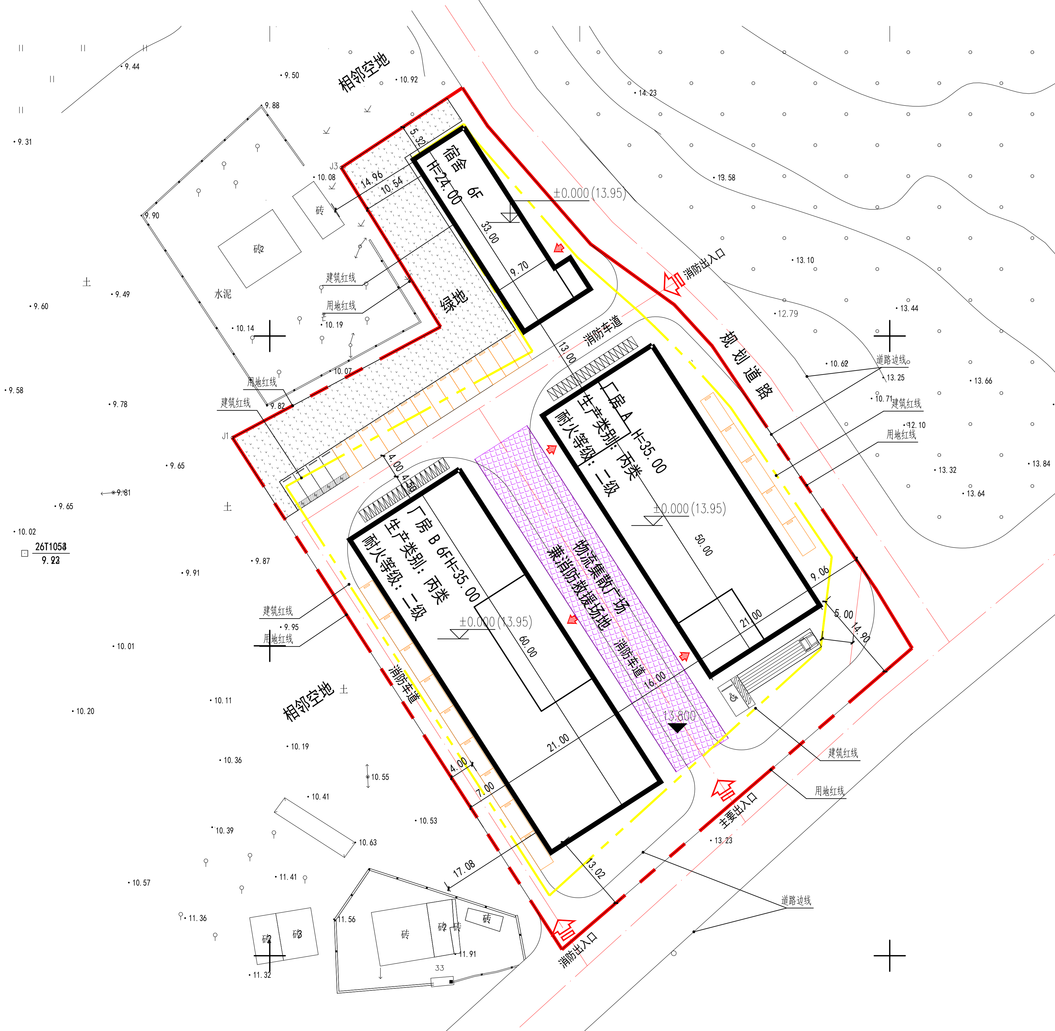
规划总平面图 1:500
