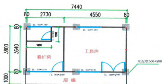
2K*4K*3P(平面图)
