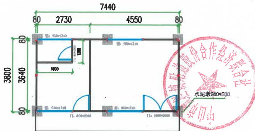
2K*4K*3P(平面图)
