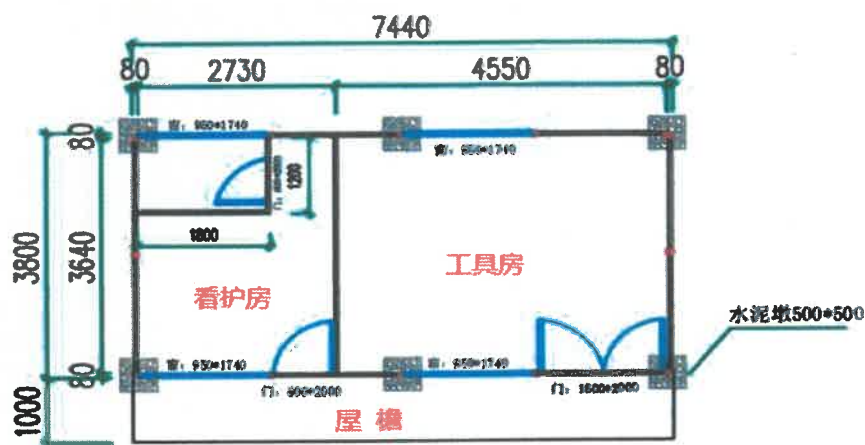
2K*4K*3P(平面图)
