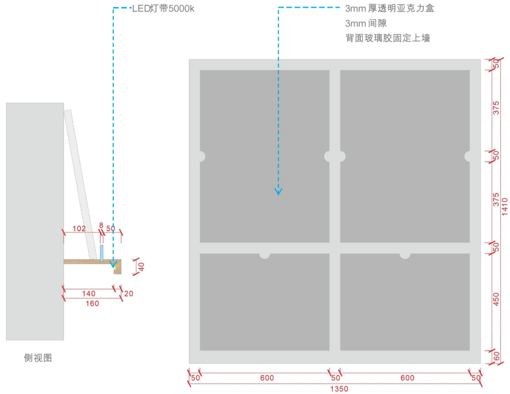
海报活动宣传亚克力展示盒尺寸图
