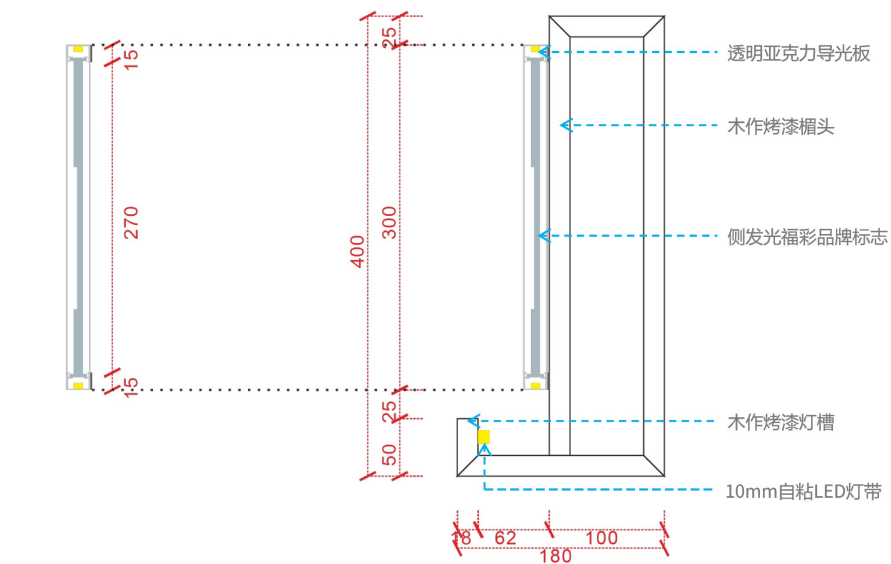
400mm高烤漆板造型门头剖面尺寸图
