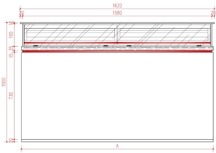
正立面图
