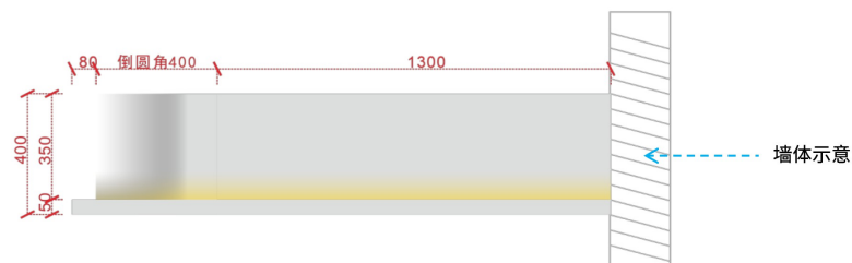
400mm高烤漆板造型门头长度尺寸规范示意图（中岛式放置）
