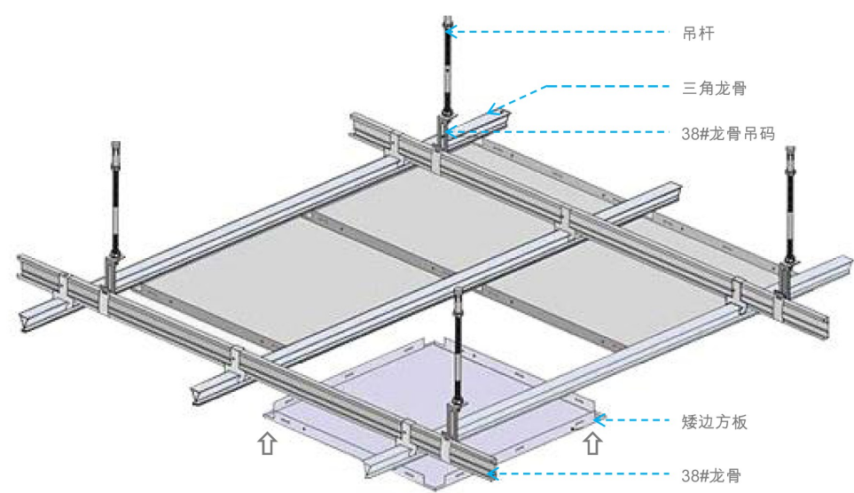
铝扣板吊顶工艺示意
