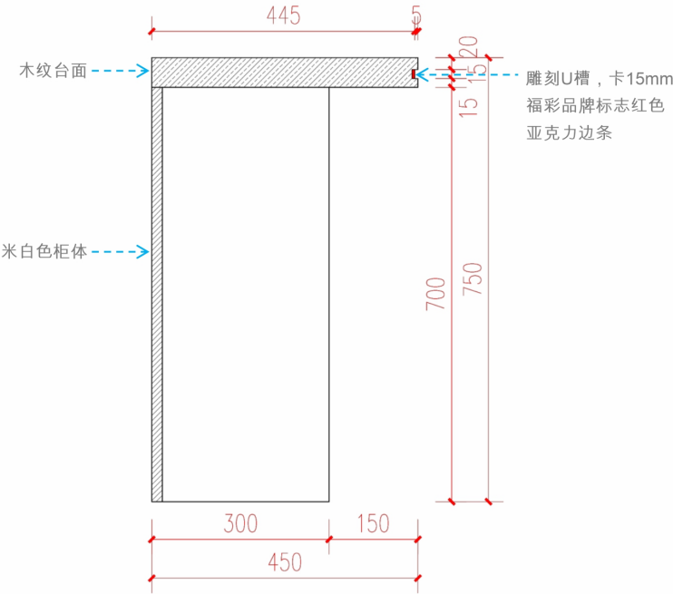
B2配套独立桌剖面图
