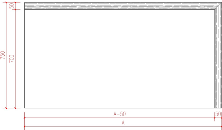
背立面图
