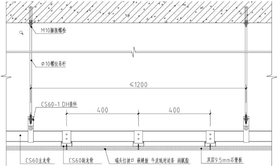
石膏板吊顶工艺示意
