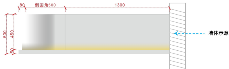
500mm高烤漆板造型门头长度尺寸规范示意图（靠墙放置）
