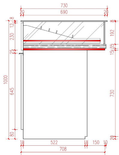
左侧视图
