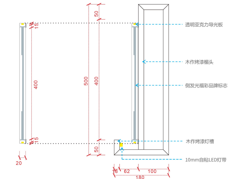
500mm高烤漆板造型门头剖面尺寸图
