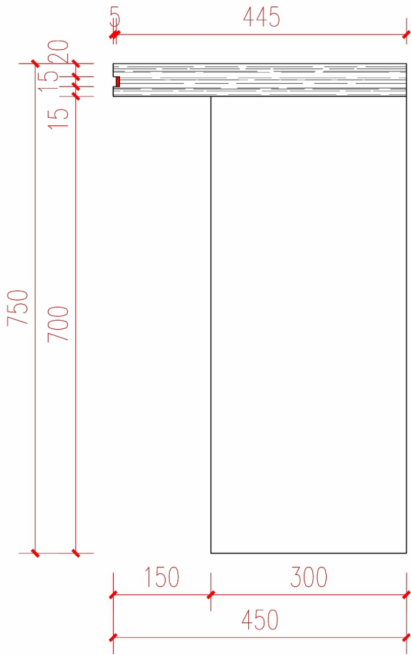
右侧视图
