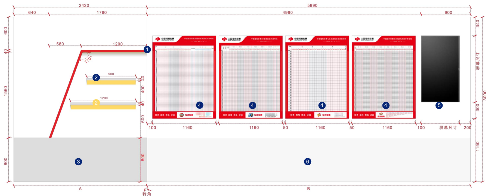
正窄右宽“L”型转角体验区墙面
