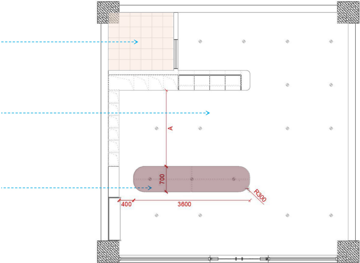
当有卫生间时，卫生间吊顶为300mm*300mm 白色铝扣板集成吊顶
