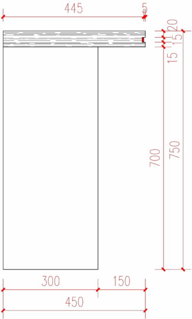
左侧视图
