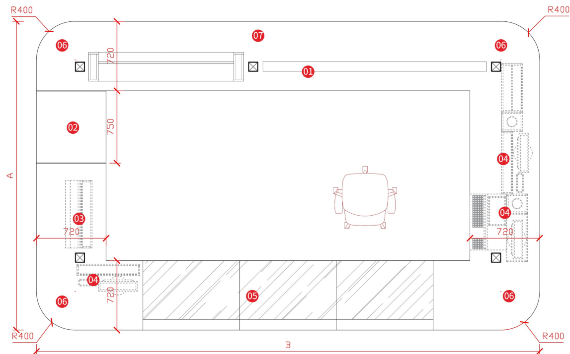
“U”型岛型店平面图
