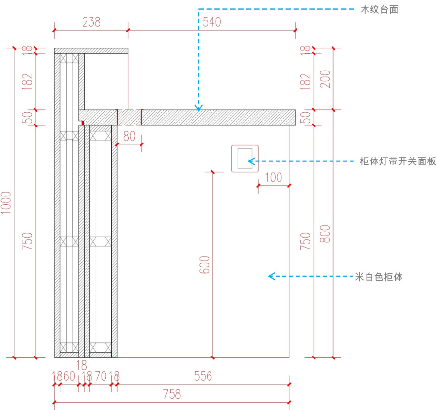
A1服务台主展柜桌面剖面图
