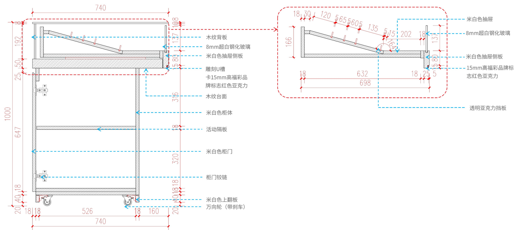
可移动展示柜剖面图
