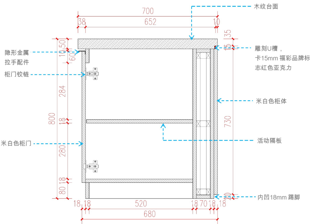
A1服务台主展柜桌面剖面图
