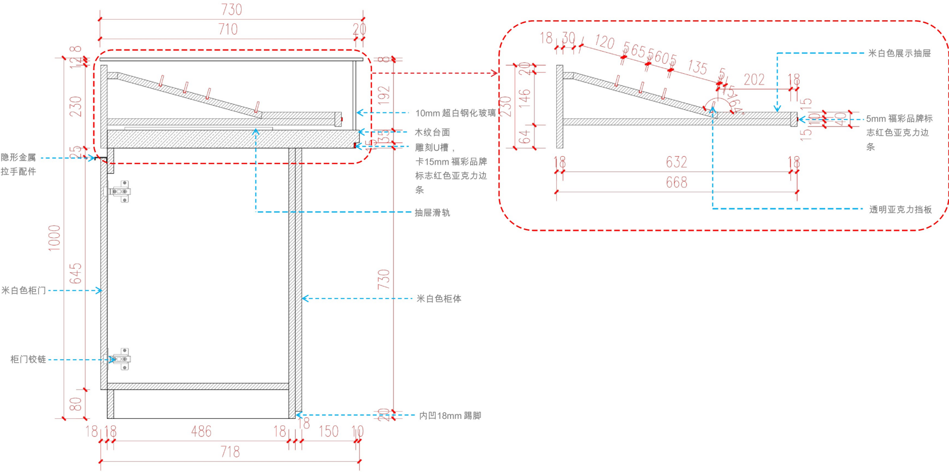
A2即开票抽屉柜剖面图
