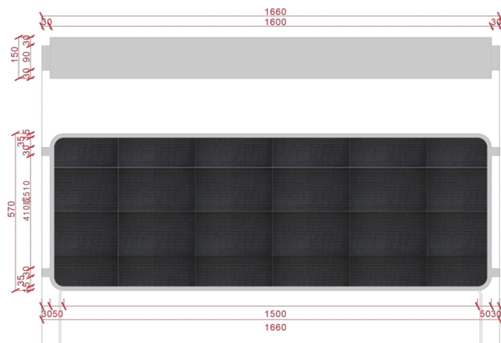
定制双面LED屏幕模块尺寸规范（建议清晰度为P2.0）
