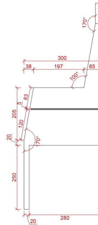
侧视图
