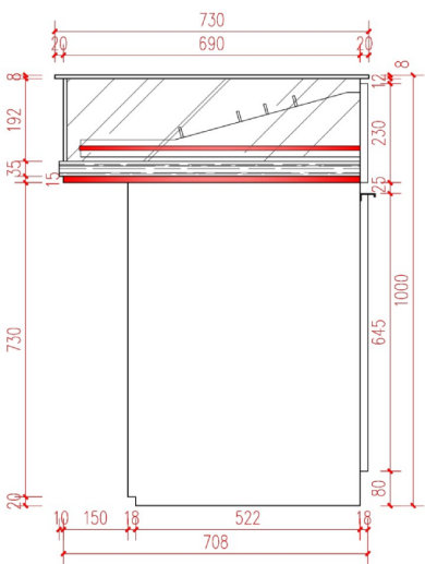
右侧视图
