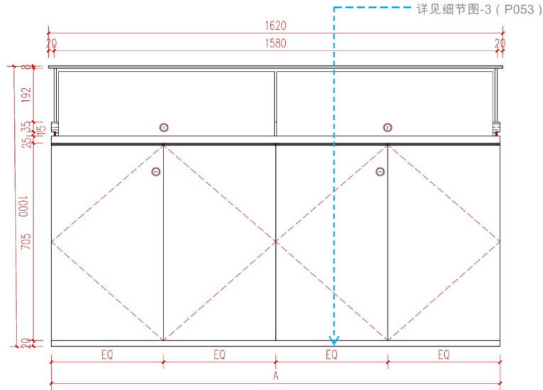
背立面图
