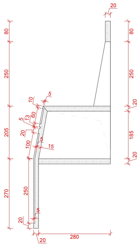
侧视结构图
