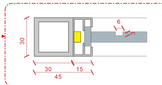
定制8mm宣传语透明导光板模块连接细节剖面图
