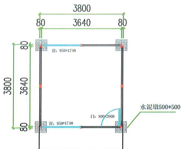
2K*2K*3P (平面图)
