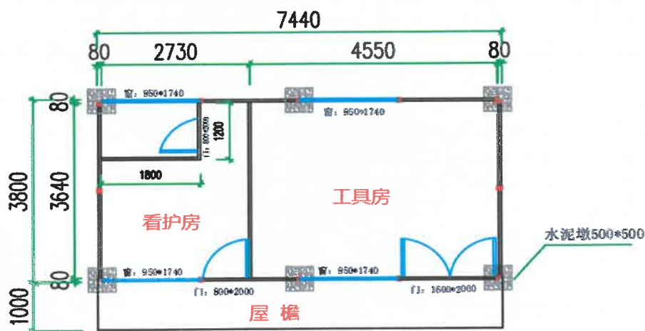
2K*4K*3P(平面图)
