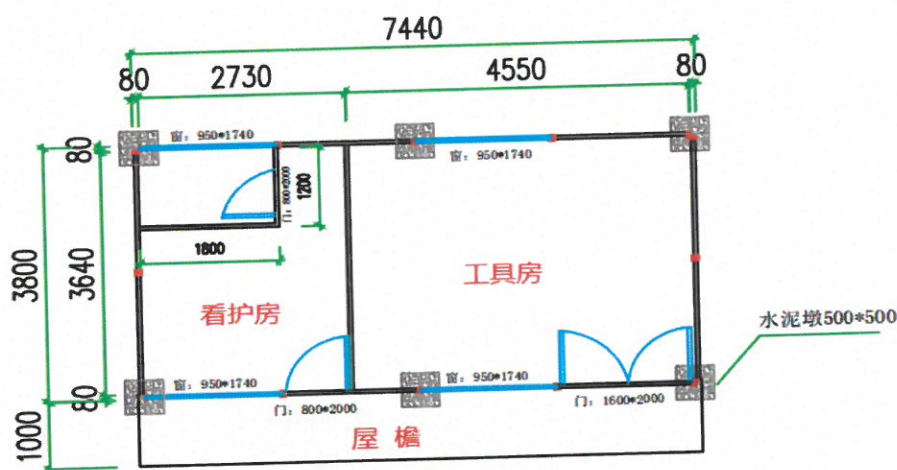
2K*4K*3P(平面图)
