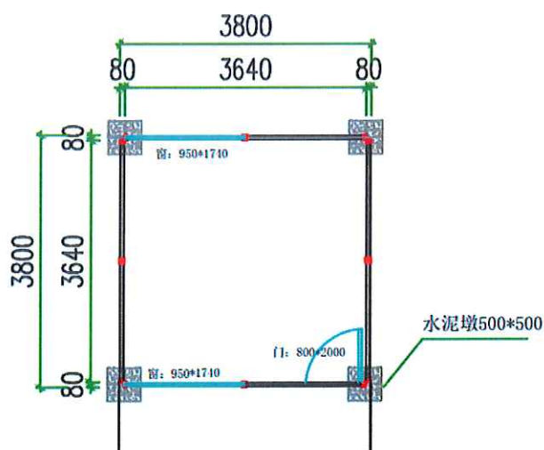
2K*2K*3P (平面图)
