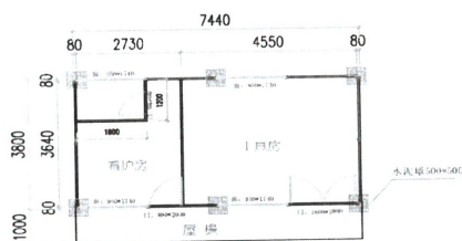
2K*4K*3P (平面图)
