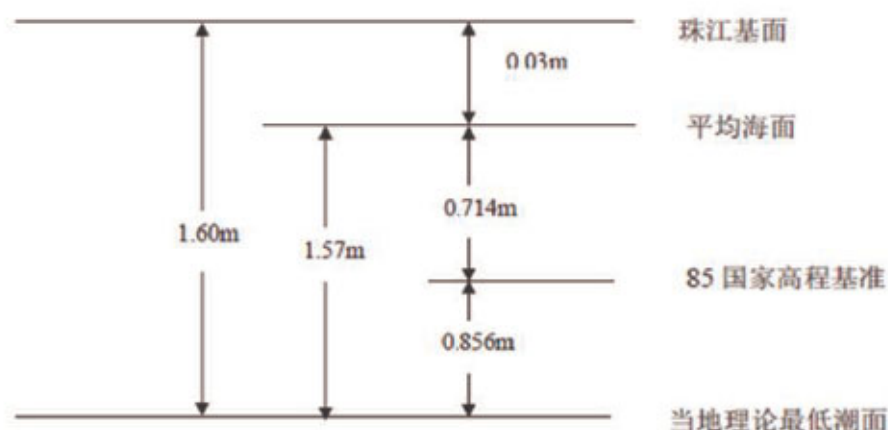
图 2.2.2-1 基面关系
