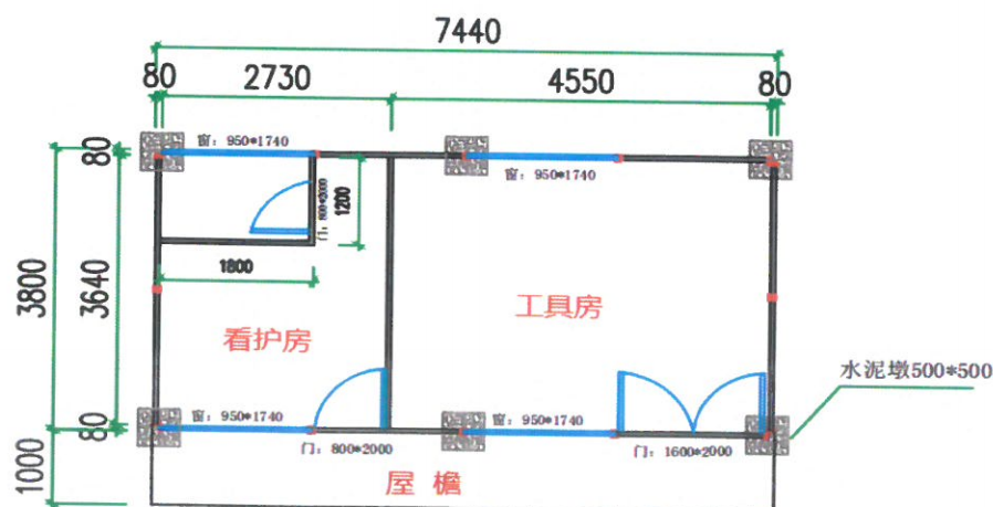
2K*4K*3P(平面图)
