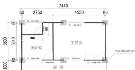
2K*4K*3P(平面图)
