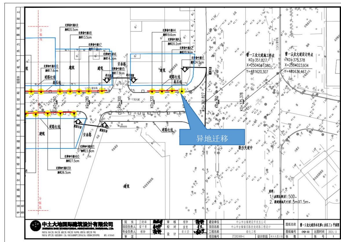
分区三迁移平面图
