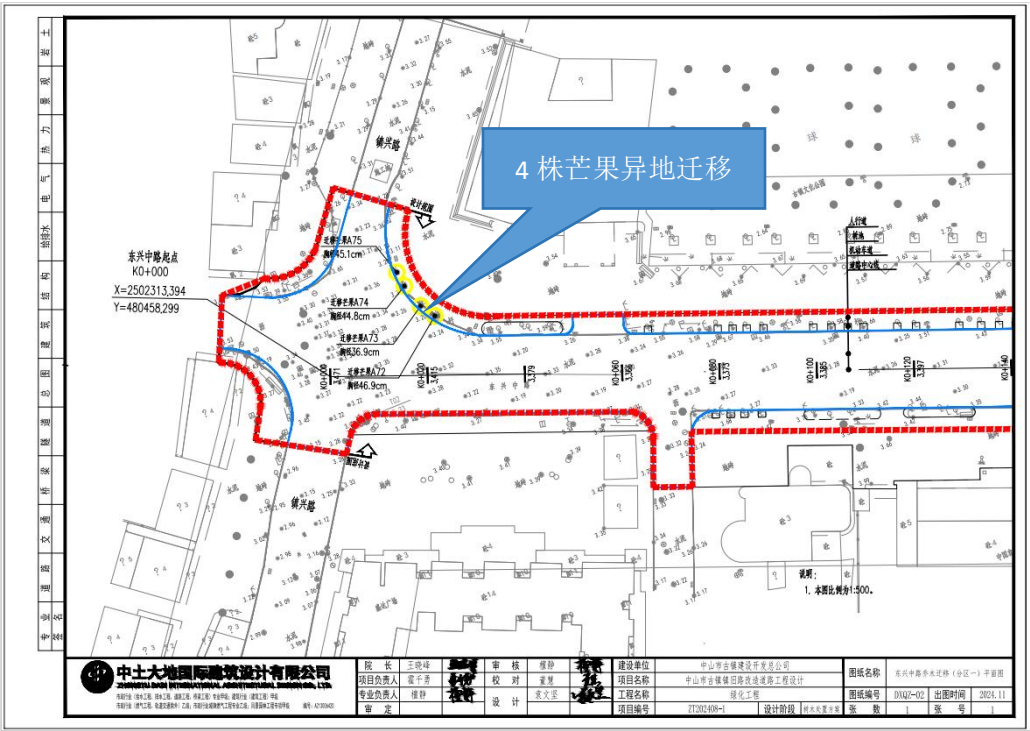
分区一迁移平面图
