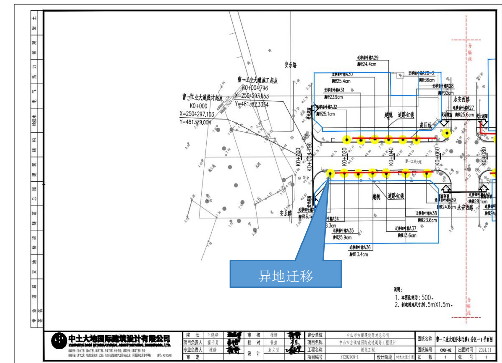
分区一迁移平面图
