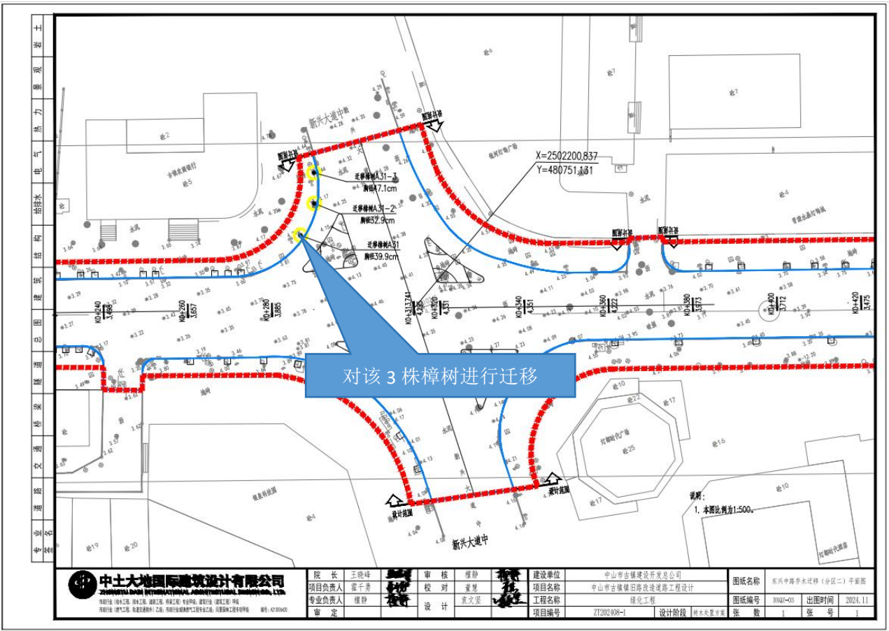
分区二迁移平面图
