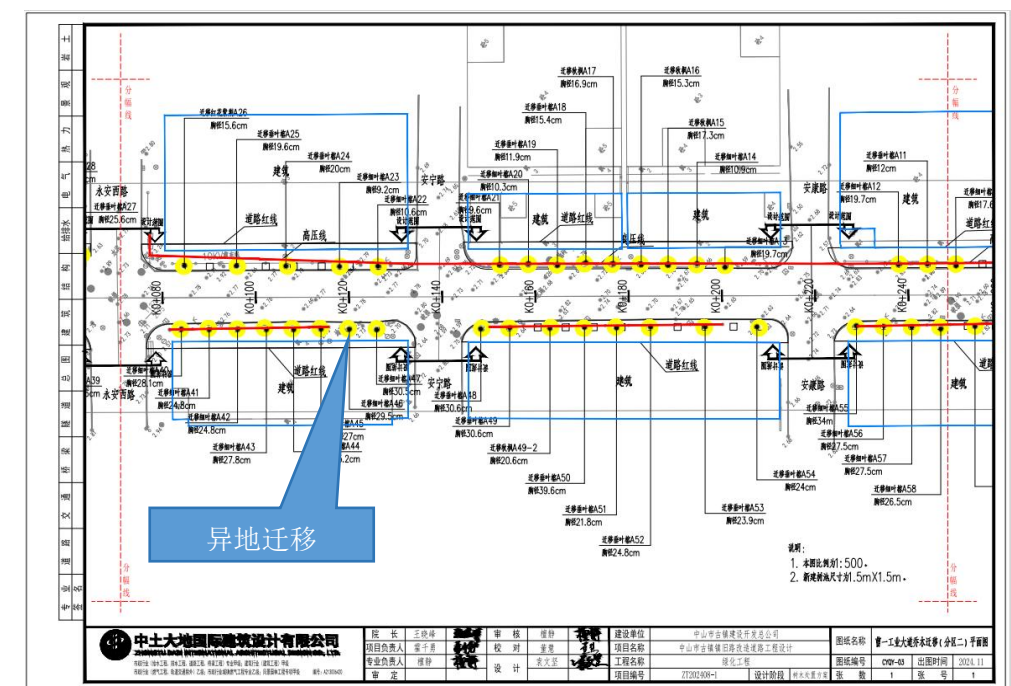
分区二迁移平面图
