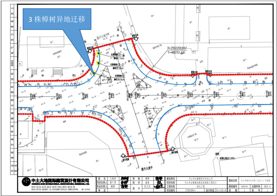
分区二迁移平面图
