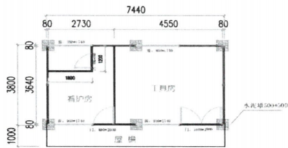
2K*4K*3P (平面图)
